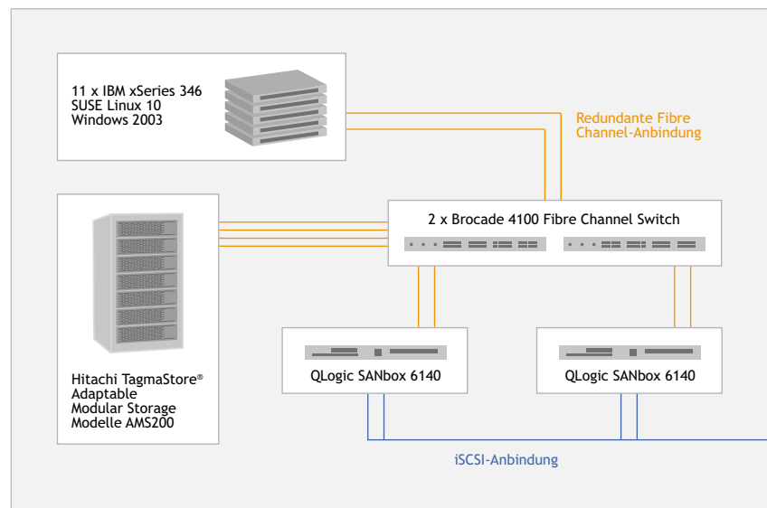
Abb.: Schematische Darstellung der SAN Infrastruktur
